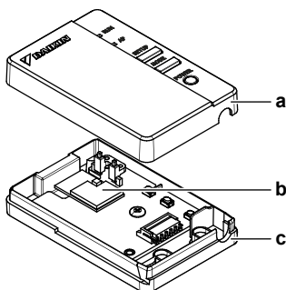
a Горно куќиште b Печатена плоча на безжичниот ЛАН-адаптер c Долно куќиште
